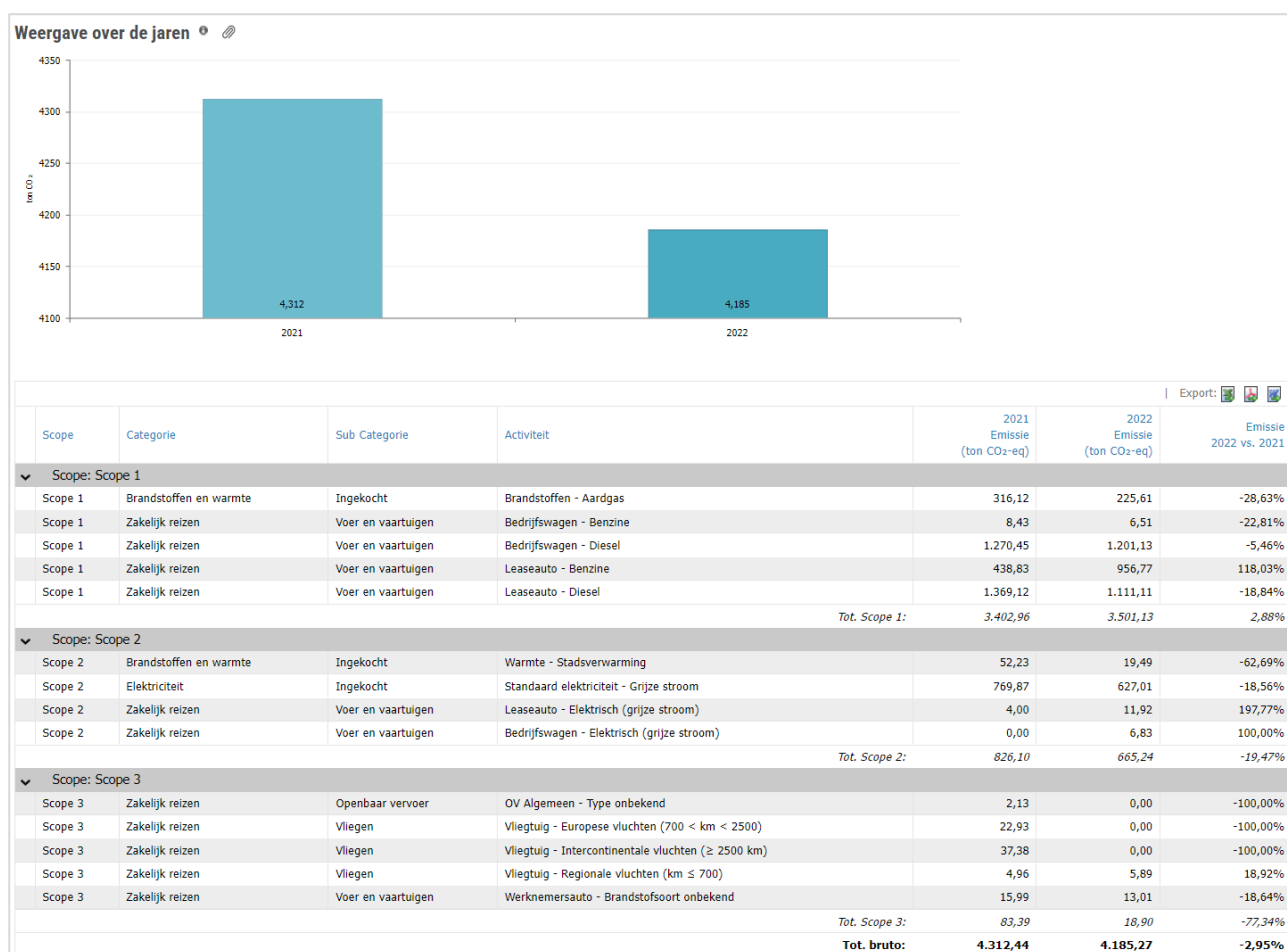
Figuur 4. CO 2 -emissies over de jaren.
