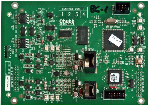
Carte UAI 2B directe IN
