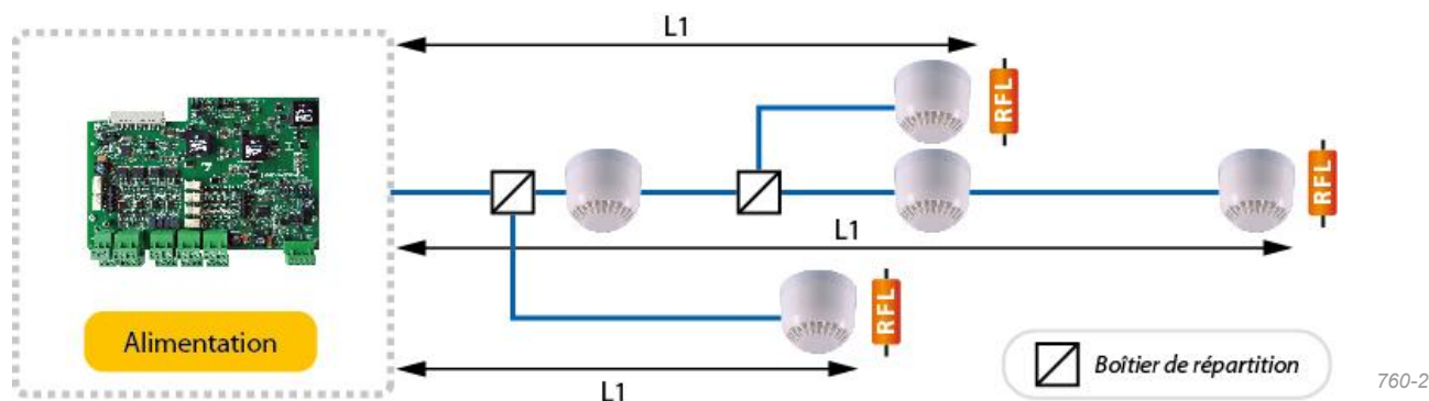
Carte UES générale / carte 4/8 voies CAN
