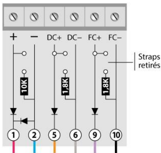
Schéma pour un DAS intermédiaire
