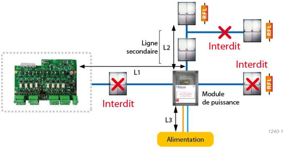
Carte UES générale / carte 4/8 voies CAN
