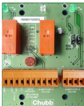
Module de puissance Image S200
